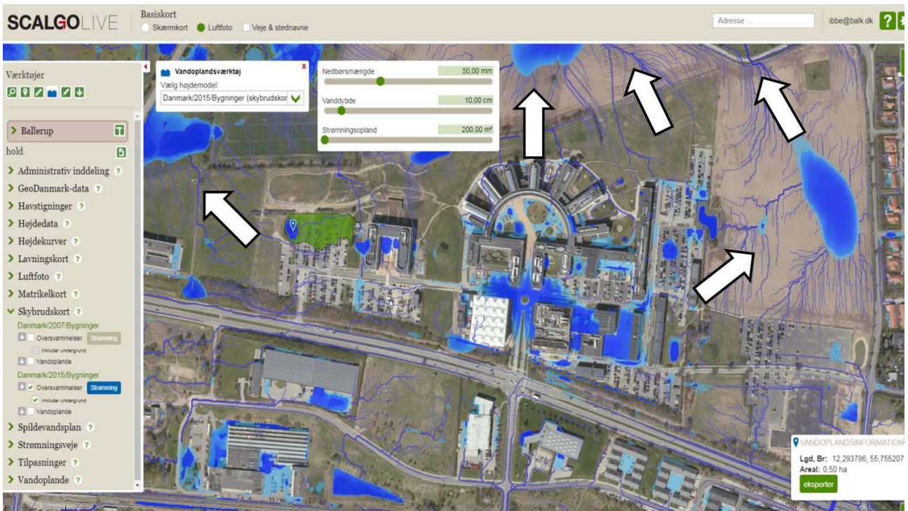
'Scalgo-model' der viser strømme og opstuvninger i området ved en 100 års regnhændelse.
