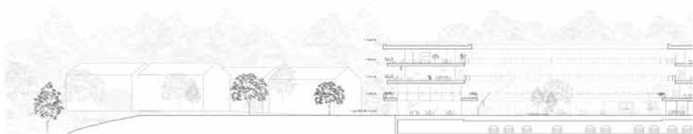
Schnitt Ost - West | 1:100
