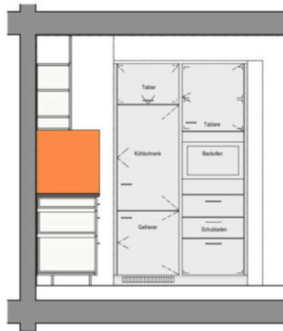
Ansicht Küche
