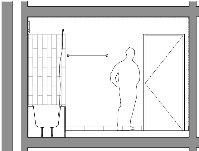
Ansicht Bad
