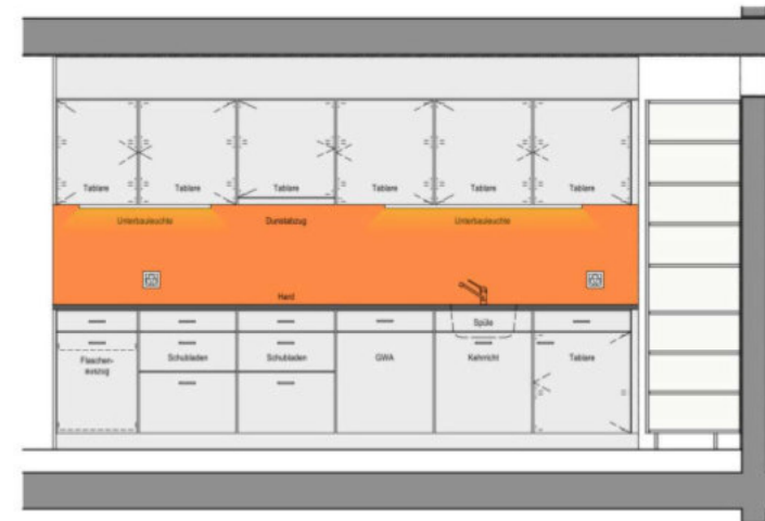
Ansicht Küche
