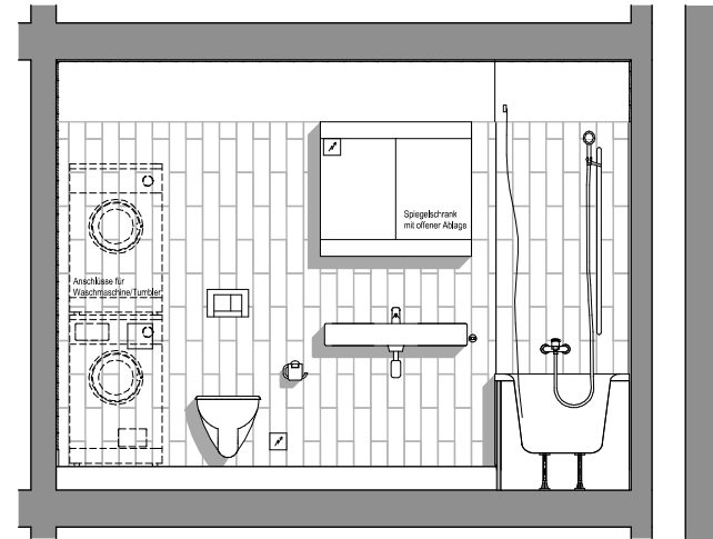
Ansicht Bad
