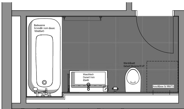
Grundriss Bad
