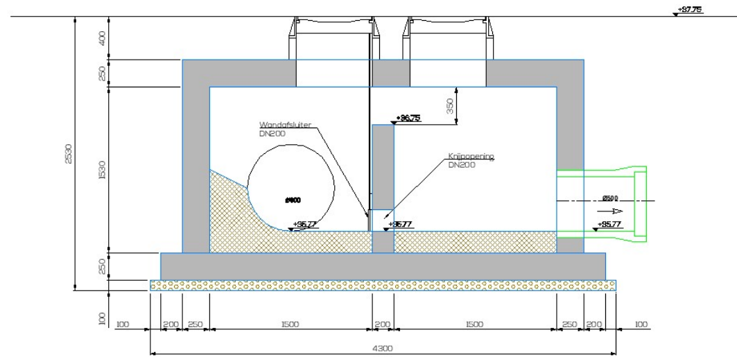
Snede A-A'
