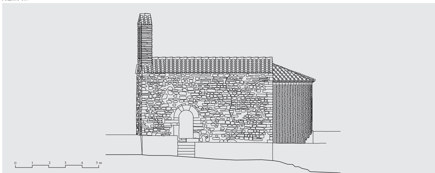
Alzado sur
